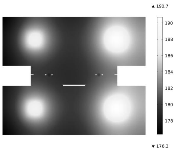
Рис. 6.6. Температурные поля: а – четверти моделируемой системы; б – поперечного сечения системы
