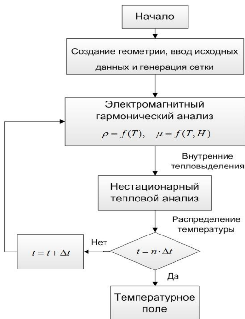
Рис. 6.1. Алгоритм связанного анализа расчёта устройств индукционного нагрева
