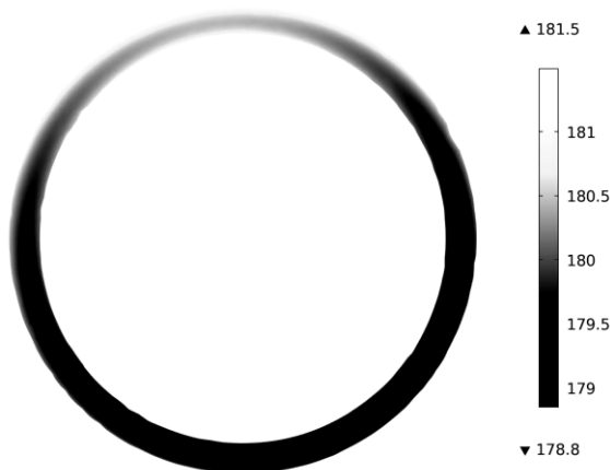
Рис. 6.7. Температурное поле продольного сечения резинового кольца
