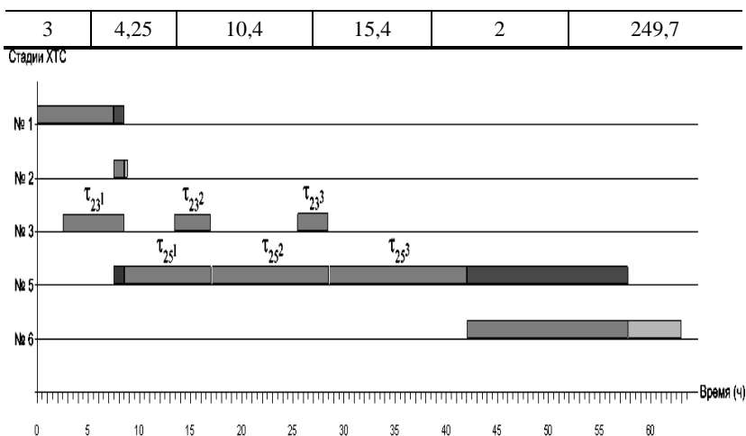
Рис. 2.3. Диаграмма цикла работы ХТС при выпуске продукта № 2
