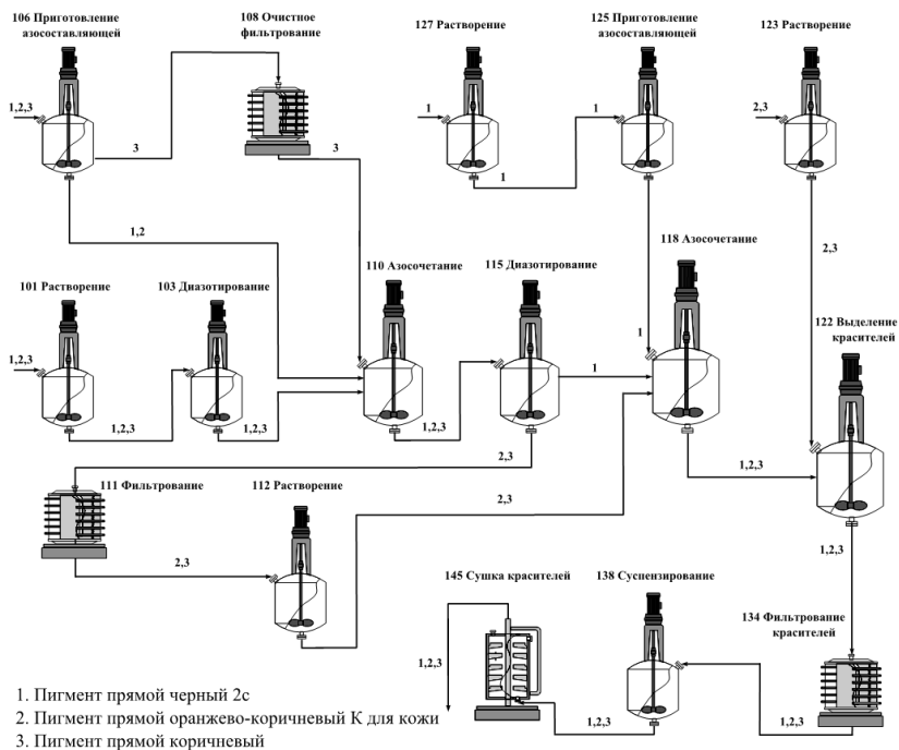
Рис 3.2. Тестовый пример химико-технологической системы 3.1. Решение задачи выбора АО для тестовой ХТС
