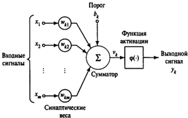
Рис. 1.1. Модель нейрона
