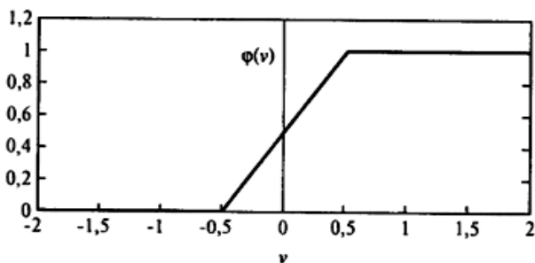
Рис. 1.3. Кусочно-линейная функция
