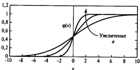
Рис. 1.4. Сигмоидальная функция для различных значений параметра a
